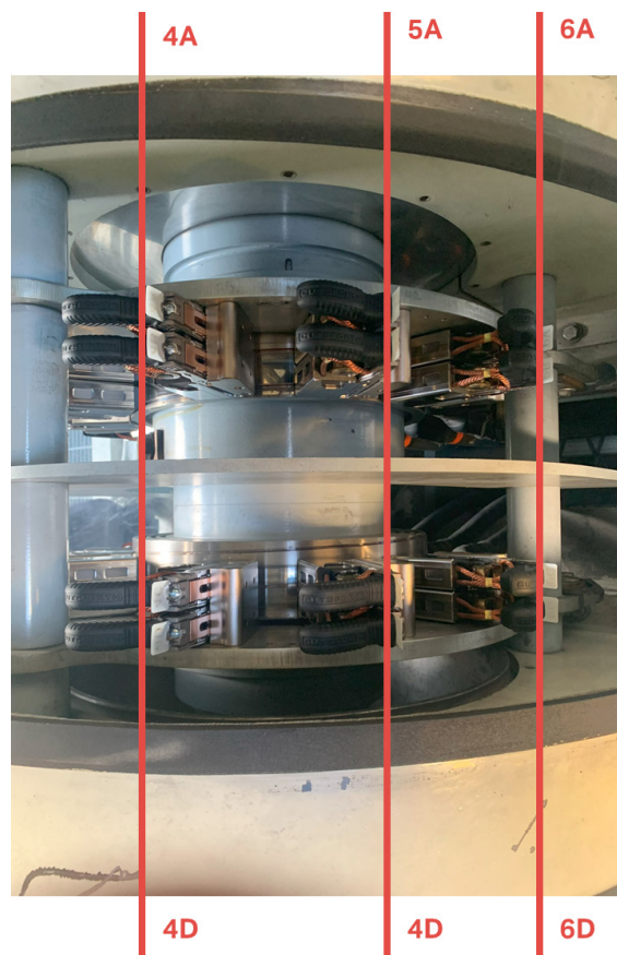
Lateral del generador
